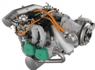
912 - Rotax 912 ULS 2 incl. optionaler Zubehör
