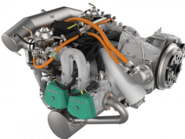
912 S 2 incl. optionalem Zubehör
